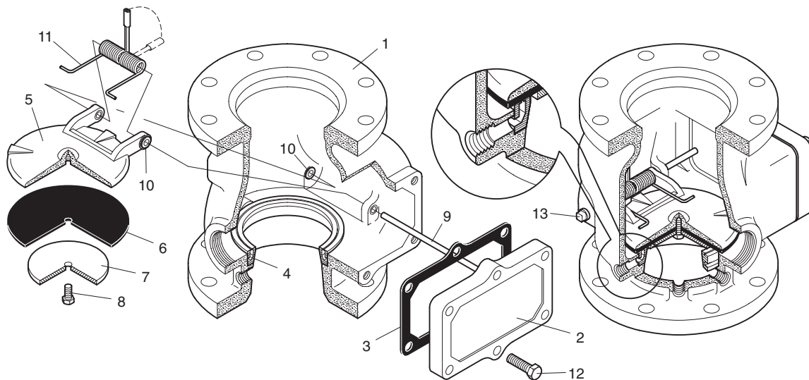
РИС. 1 СИГНАЛЬНЫЙ КЛАПАН DN100, DN150 и DN200, МОДЕЛЬ AV-1-300 —СБОРКА—
