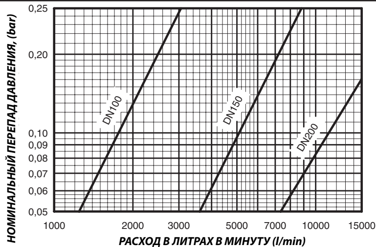
РИС. 2 СИГНАЛЬНЫЙ КЛАПАН DN100, DN150 и DN200, МОДЕЛЬ AV-1-300 — НОМИНАЛЬНАЯ ПОТЕРЯ ДАВЛЕНИЯ В ЗАВИСИМОСТИ ОТ ПОТОКА —
