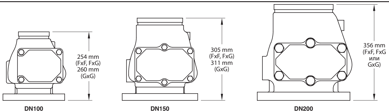
РИС. 3 СИГНАЛЬНЫЙ КЛАПАН DN100, DN150 и DN200, МОДЕЛЬ AV-1-300 — ВНЕШНИЕ РАЗМЕРЫ —
